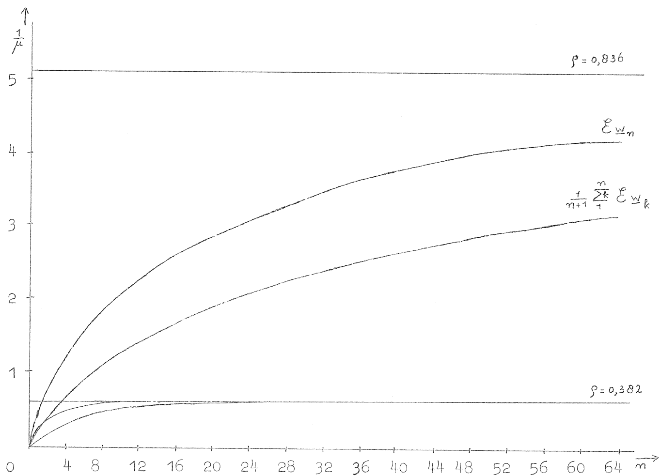
Fig. 11. E_{w_n} en \frac{1}{n+1} \sum_{k=0}^n E_{w_k} bij exponentiële bedienings- tijden als functies van n voor \rho = 0,382 , \rho = 0,836 , ( E_s = 1 ).
