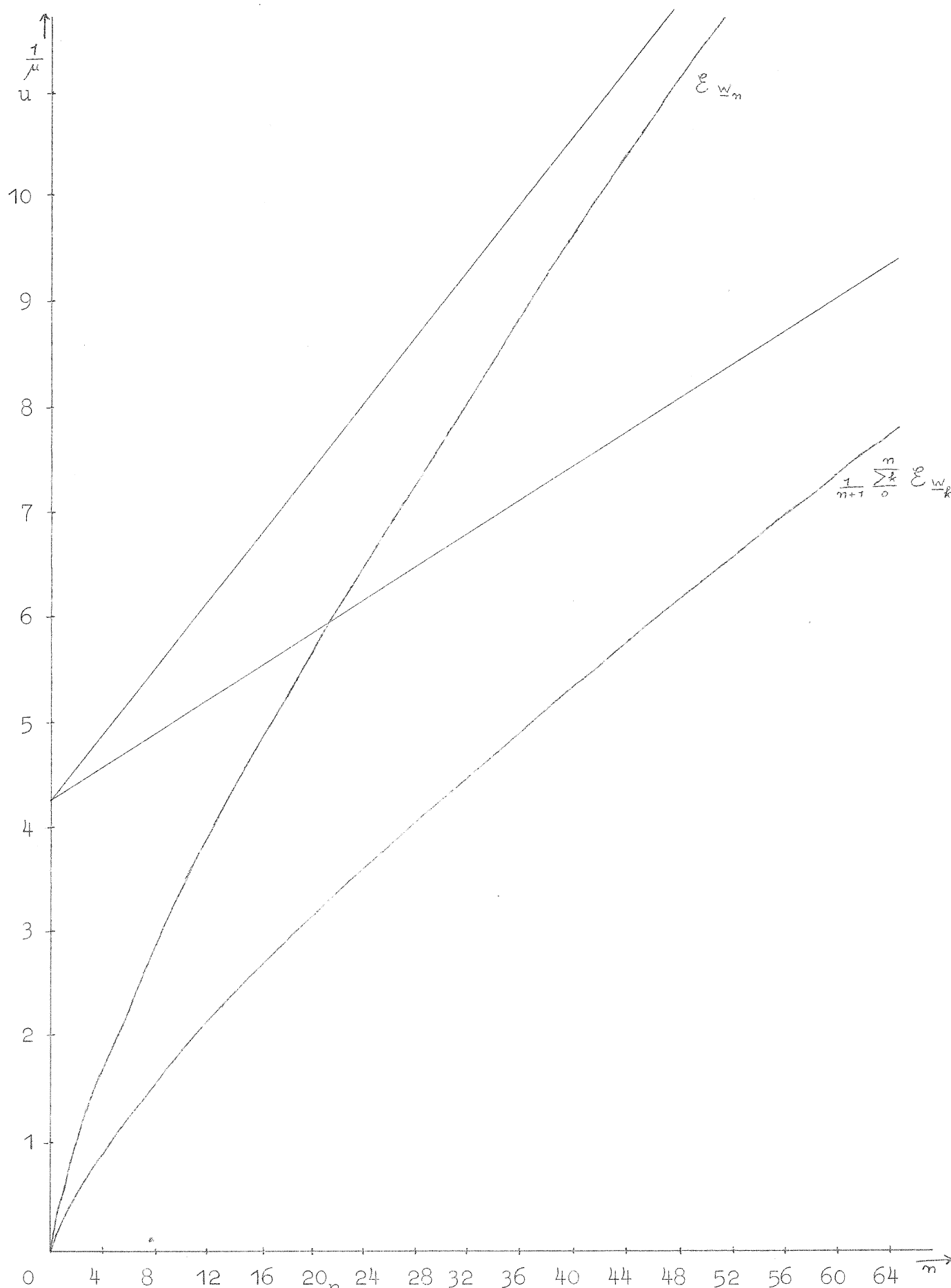
Fig. 12. \xi_{w_n} en \frac{1}{n+1} \sum_{k=0}^n \xi_{w_k} als in fig. 11 voor \rho = 1,196 en de
