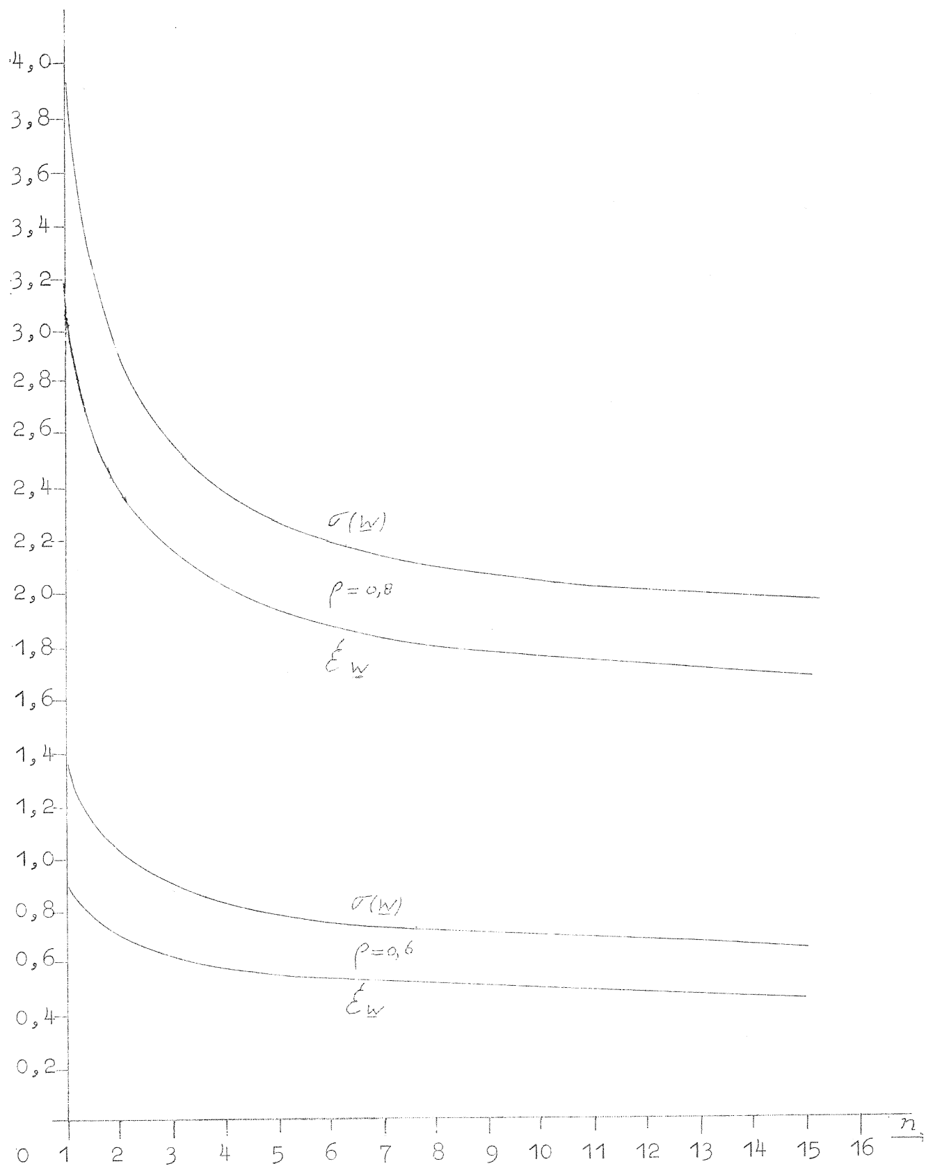
Fig. 10. Gemiddelde E \underline{w} en spreiding \sigma(\underline{w}) van de wachttijdverdeling bij een gamma verdeling met n vrijheidsgraden voor de bedieningstijd als functie van n .
